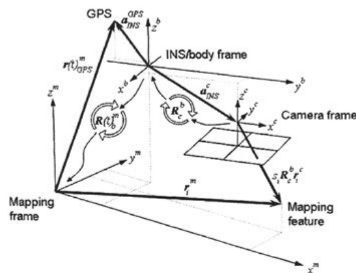
شکل ۱: زمین مرجع سازی مستقیم
